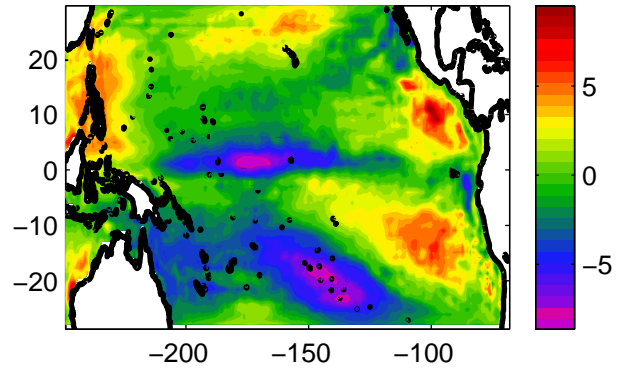
T-MODE SST EOF 3 7.472%
