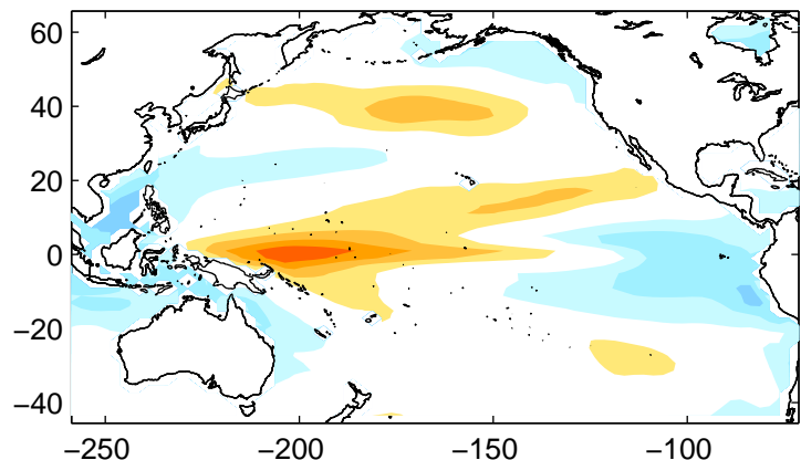
M3 Pacific SST EOF-2
